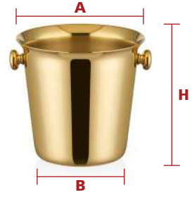
MİNİ BUZ KOVASI KONİK NO:1 MINI ICE BUCKET A46030.TA (Sade / Plain) A - Ø 12 cm B - Ø 9 cm H - 11 cm
